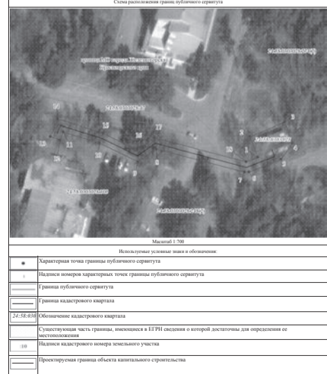
Рис. 4. Схема расположения границ публичного сервитута
